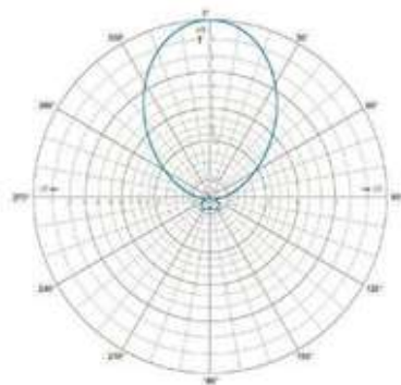
380-470MHz Horizontal Pattern
