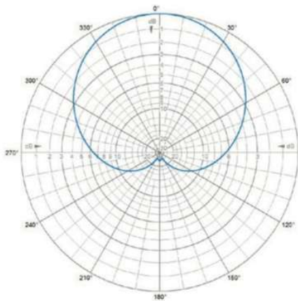
380-470MHz Horizontal Pattern
