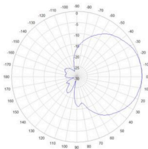
Horizontal Beamwidth
